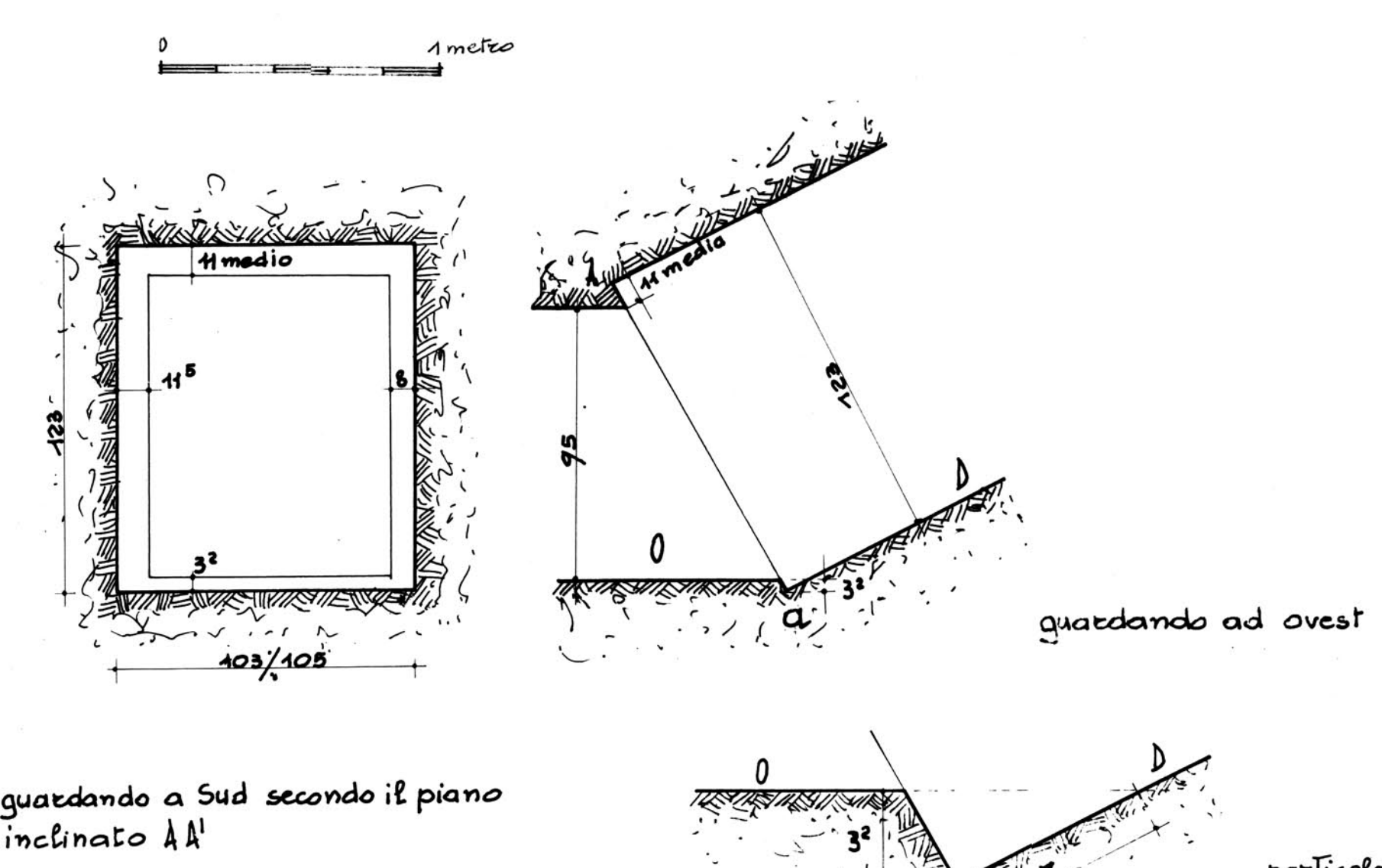
FIG. 3 PARTICOLARE DELLA SEZIONE A-a
