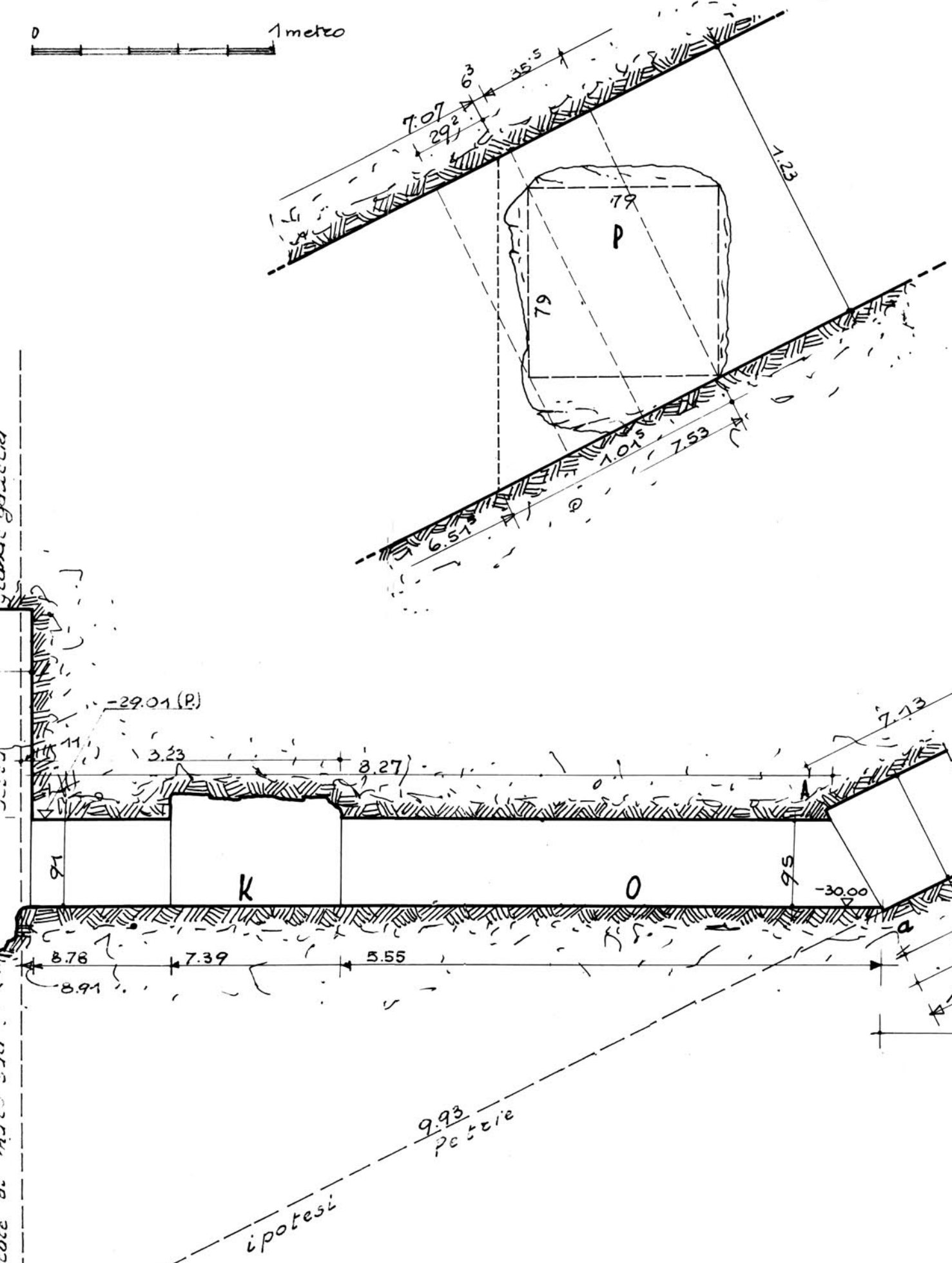
FIG. 2 PARTICOLARE DELLO SBOCCO INFERIORE DEL POZZO (Edgar)
