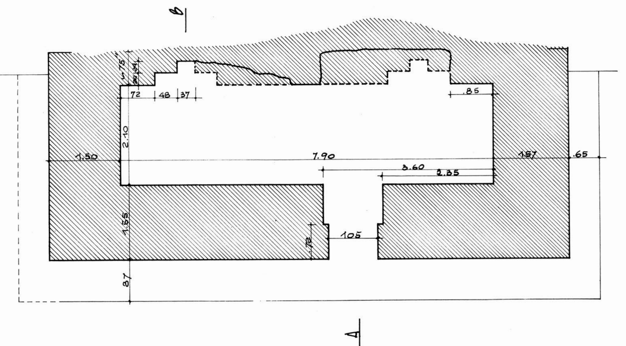
fig. 6 Pianta
