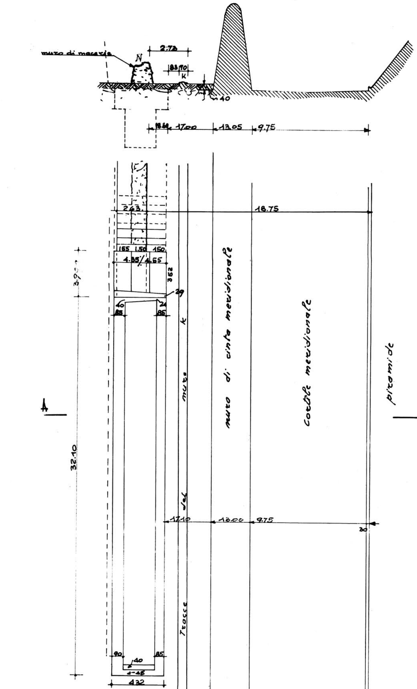
fig.9 Pianta
