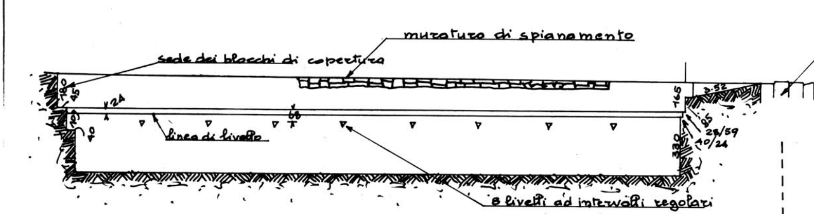
fig.11 SEZIONE J-M DEL CORTILE MERIDIONALE A W DELLE BARCHE
