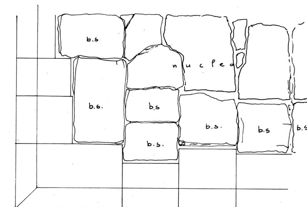
FIG. 12-13 SCHEMA DELLA DISTRIBUZIONE DEI BLOCCHI IN DUE CORSI SUCCESSIVI
