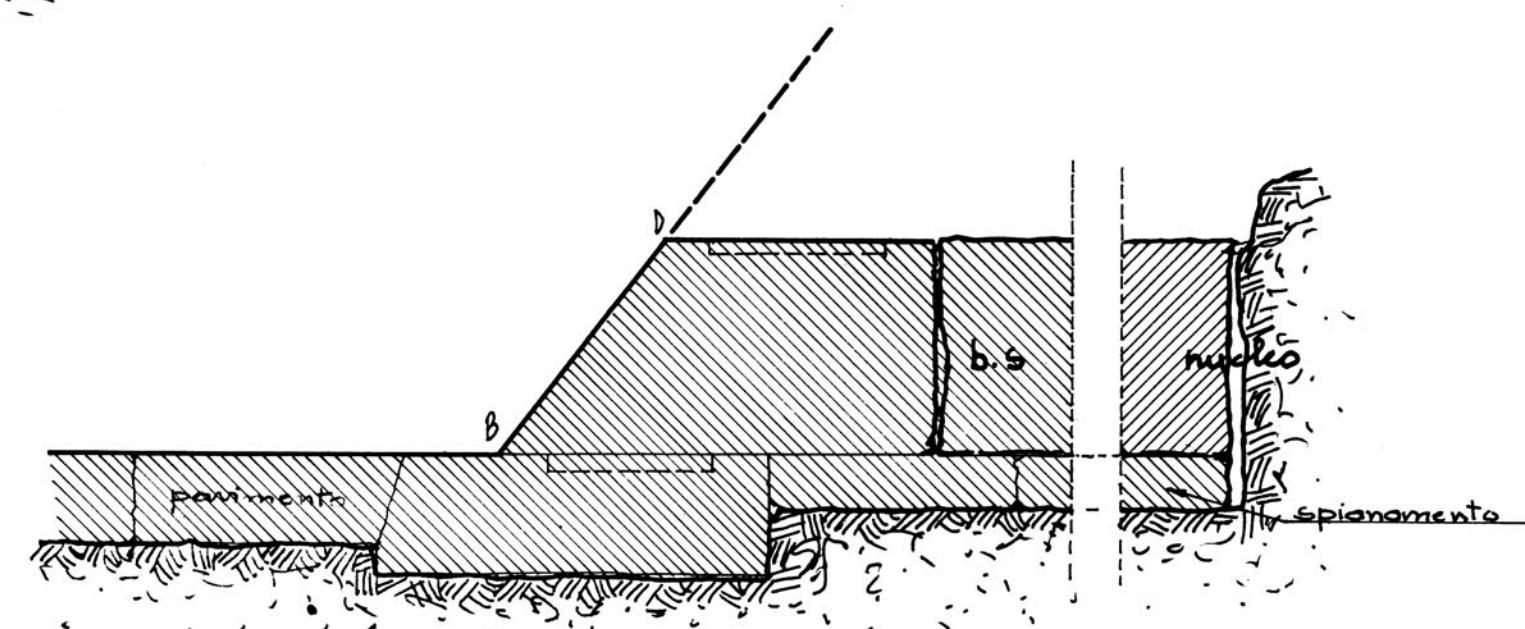
Fig. 16 Sezione AD secondo Borchardt (racc.)
