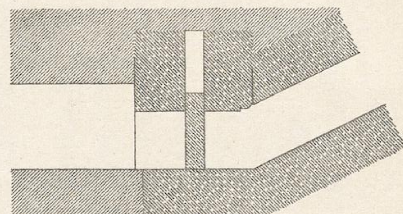
Detail b Fallsteinkonstruktion.
