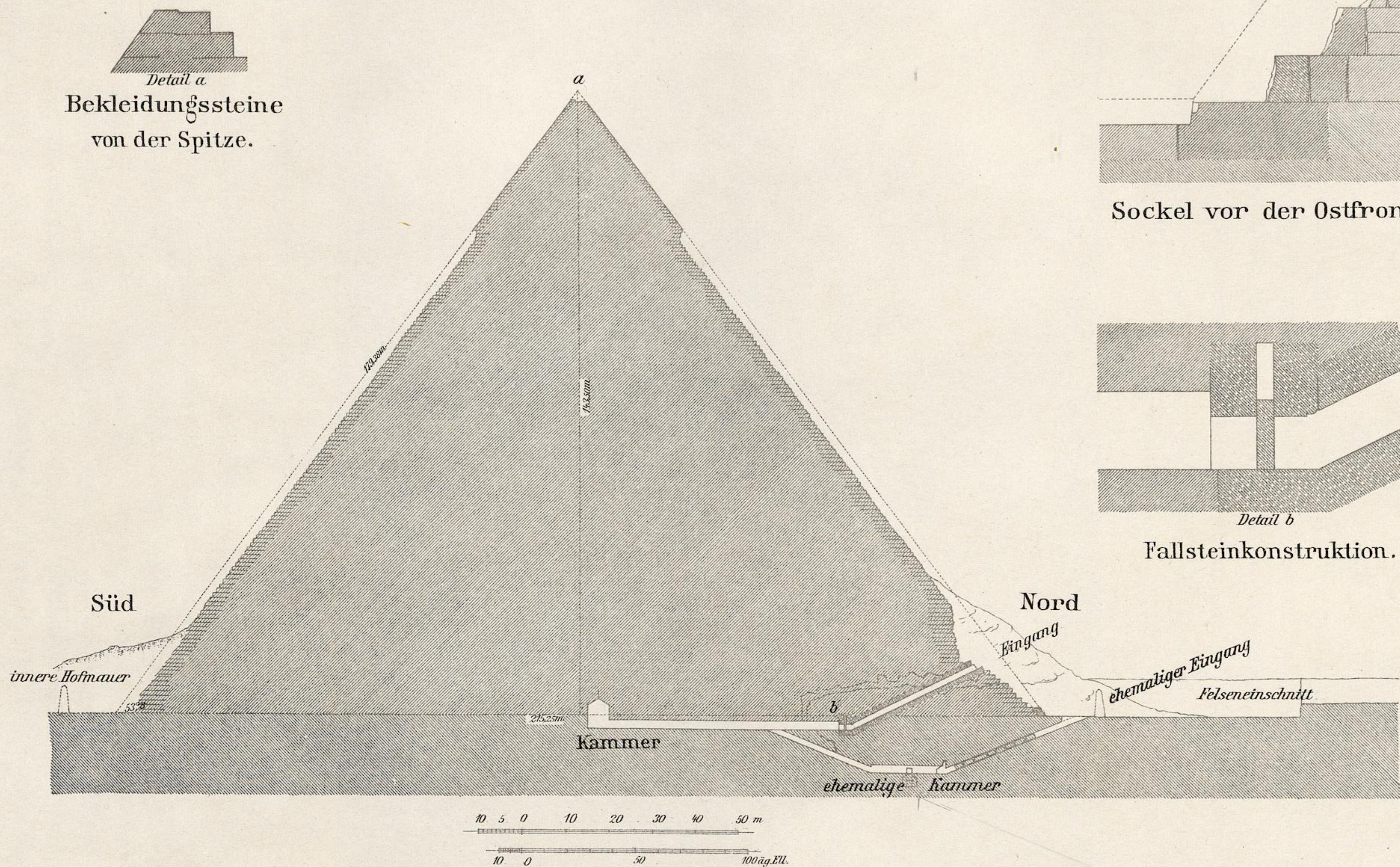
Schnitt durch die Pyramide.
