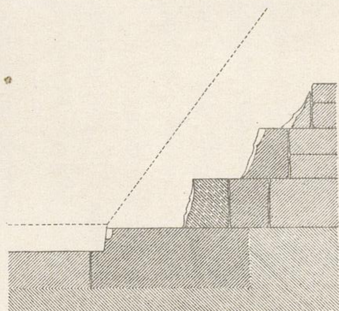
Sockel vor der Ostfront.
